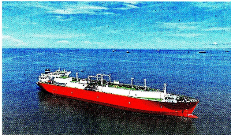
La embarcación tiene 285 metros de eslora. REGASIFICADORA DEL PACÍFICO
